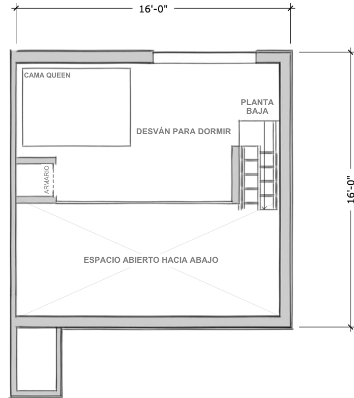
Desván para dormir: 141 pies cuadrados
