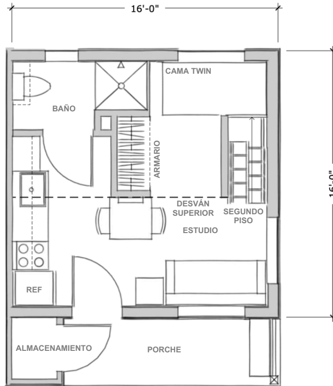
Planta baja: 262 pies cuadrados
