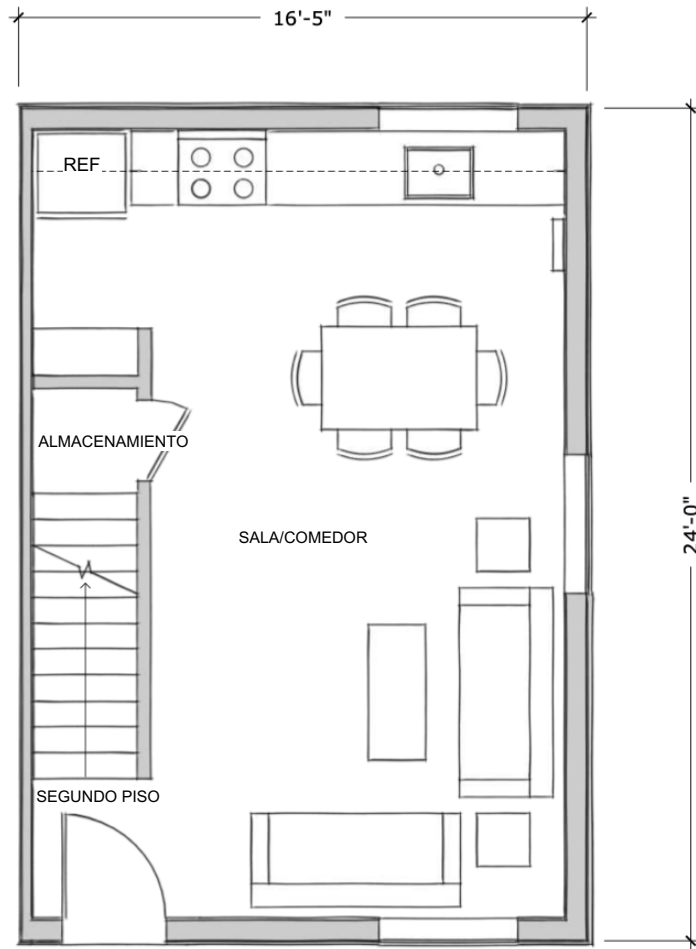
Primer piso: 394 pies cuadrados
