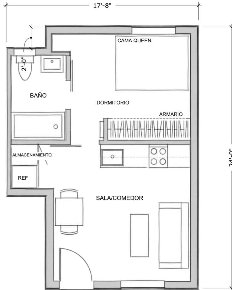
Planta baja o segundo piso: 384 pies cuadrados
