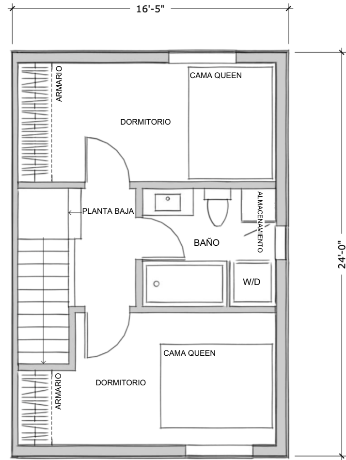
Segundo piso: 394 pies cuadrados
